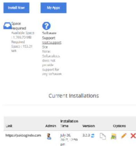
Gambar 6. Penggunaan Moodle
