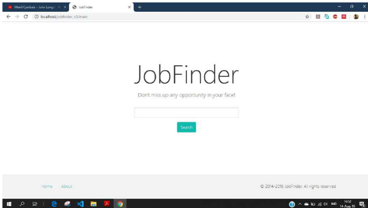
Gambar 5 Input Keyword
