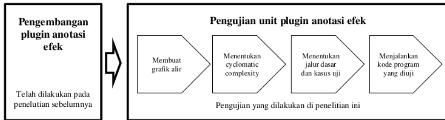
Gambar 3 Diagram alur pengujian plugin anotasi efek
