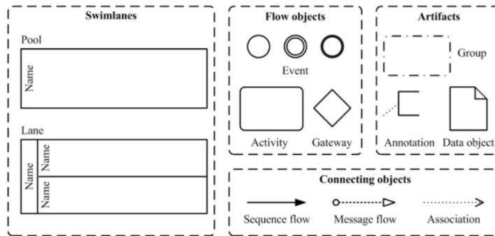
Gambar 1 Kategori dari Elemen BPMN, sumber: White (2004)
