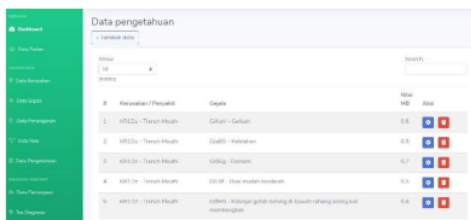
Gambar 15. Halaman Pengetahuan
