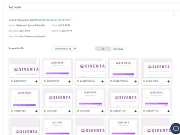
Gambar 9 Hasil Testing Compatibility Dengan LambdaTunnel
