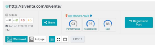
Gambar 7 Hasil Testing Dengan CrossBrowserTesting
