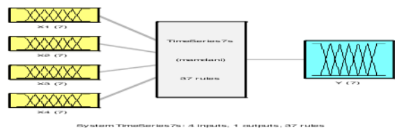
Gambar 2. Tampilan model FIS untuk 4 input, 1 output dan 7 fuzzy set.
