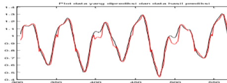
Gambar 3. Grafik output FIS dan data aktual
