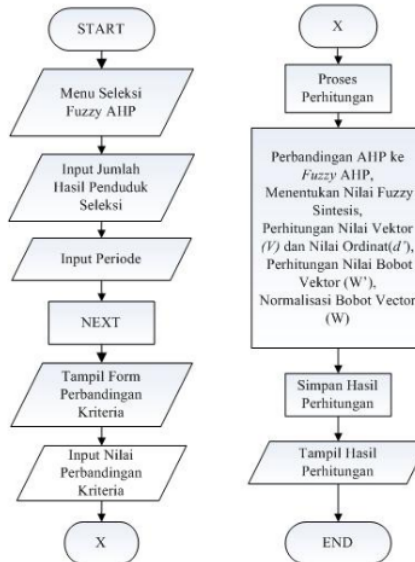
Gambar 7. Flowchart Hitung FAHP
