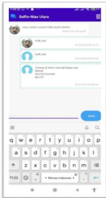
Gambar 8. Fitur Chat
