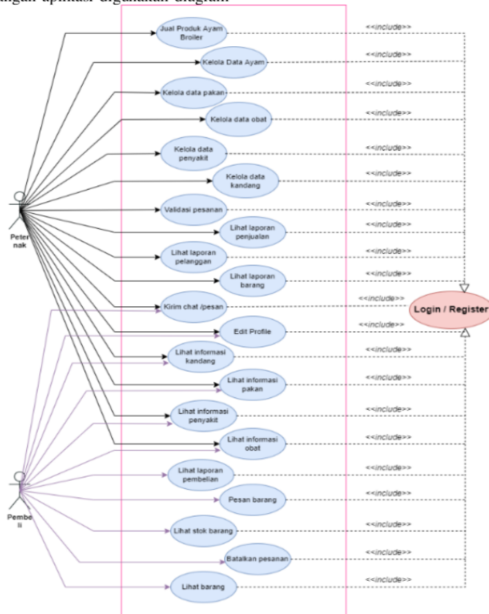
Gambar 2. Diagram Use Case Aplikasi
