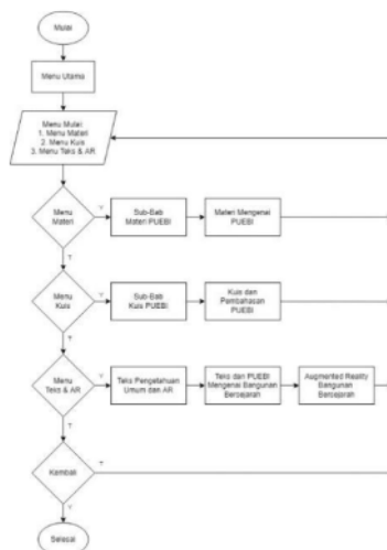
Fig 6. Menu Mulai (Start Menu) Flowchart
