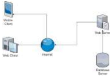
Gambar 3. Arsitektur Aplikasi
