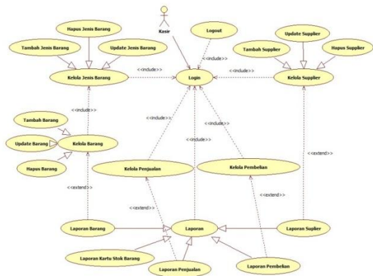
Gambar 3. Use Case Diagram Sistem Informasi Penjualan Hagas Tani
