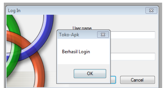
Gambar 11. Login Sukses
