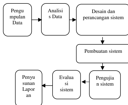
Gambar 2. Tahapan penelitian
