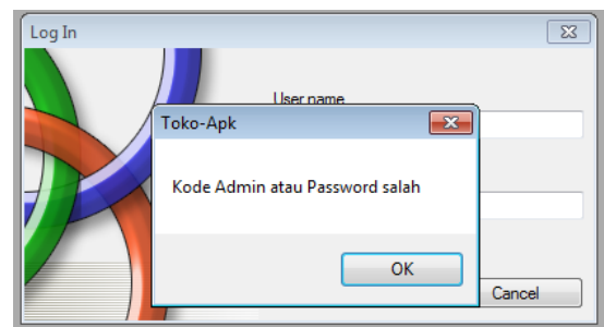
Gambar 10. Login Error
